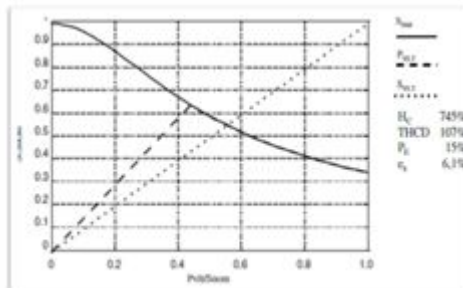
Fig. 3.2 S/Snom Vs Pv/It Snom
