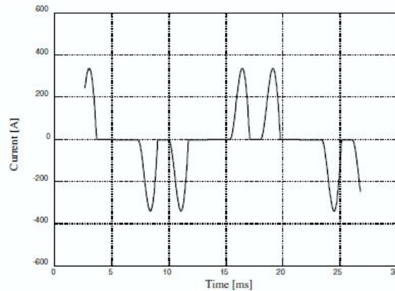
Fig. No.2.1 Actual input current
