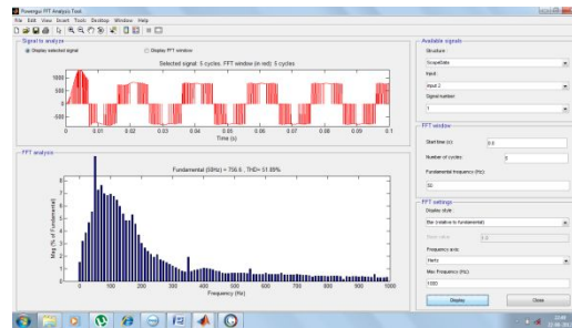
Fig. 3.7 V_{inv} -THD=51.89%
